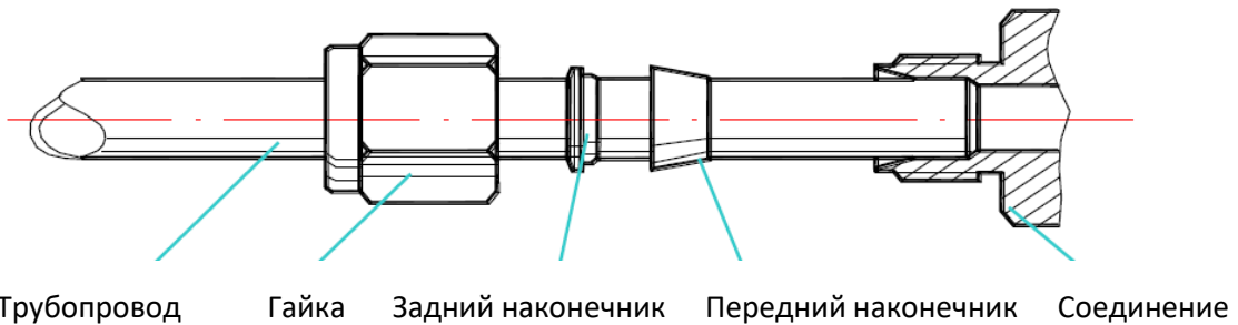
Рисунок 5. Зажимное соединение
